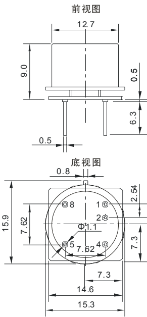
封装尺寸:
