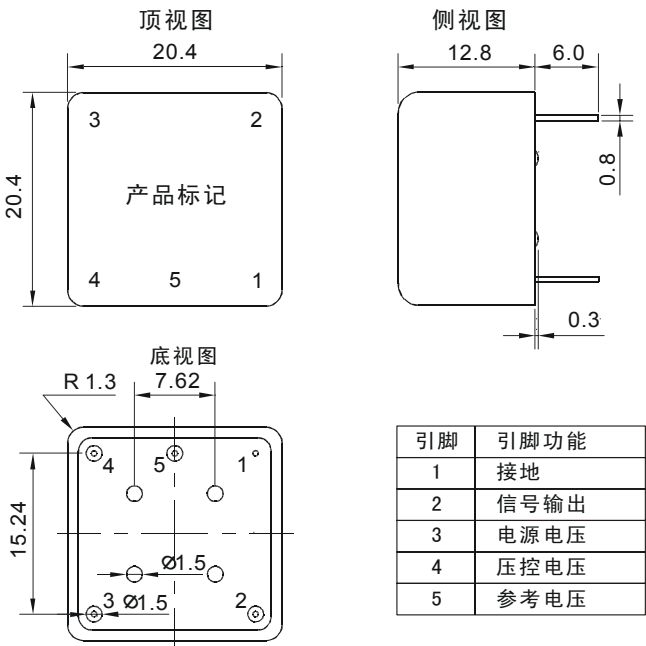
封装尺寸:
